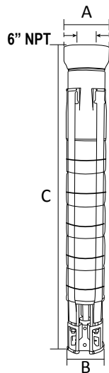
Acoplamiento NEMA 6"
