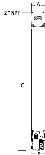
Acoplamiento NEMA 6" Fig. 3
